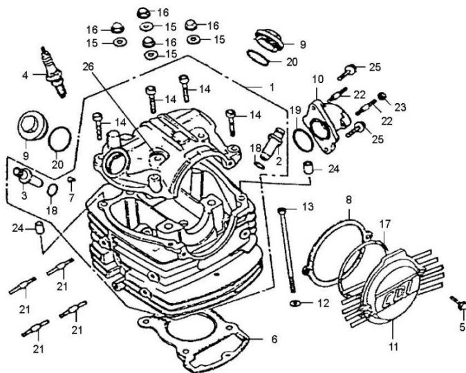
E07 = 汽缸头和盖 / CYLINDER HEAD & COVERS / CULATA Y CUBIERTAS
