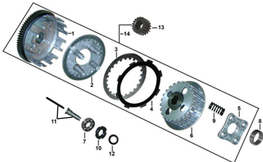
E03 = 离合器 / CLUTCH / EMBRAGUE
