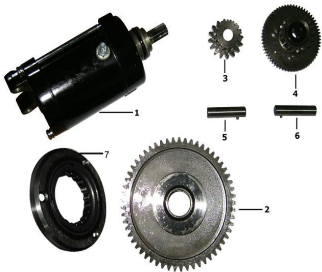
E13 = 启动马达 / STARTING MOTOR / ARRANQUE DE MOTOR
