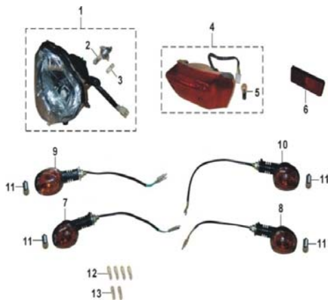
B09 = 灯具 / LIGHTS / LUCES DIRECCIONALES Y REFLEJANTES
