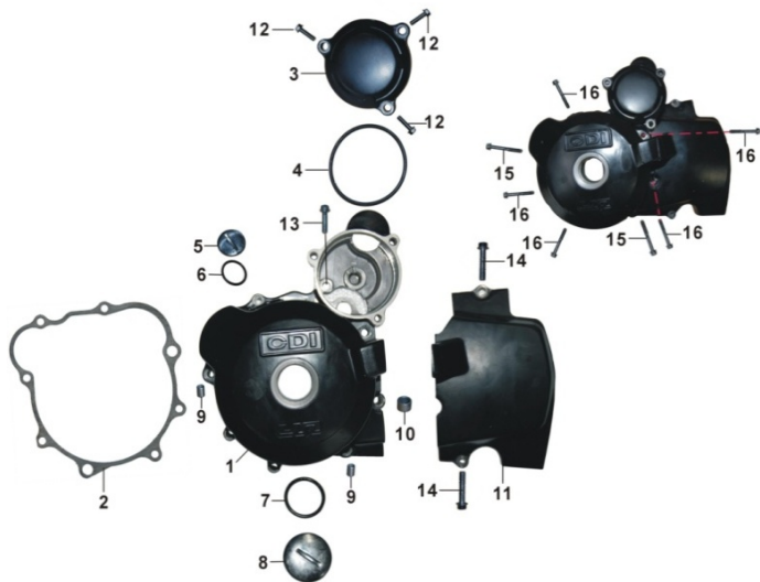
E12 = 右箱体 / RIGHT CRANKCASE COVER / CUBIERTA DERECHA DE MOTOR
