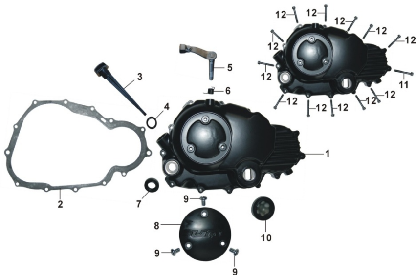
E09 = 左曲轴箱 / LEFT CRANKCASE COVER / CUBIERTA IZQUIERDA DE MOTOR
