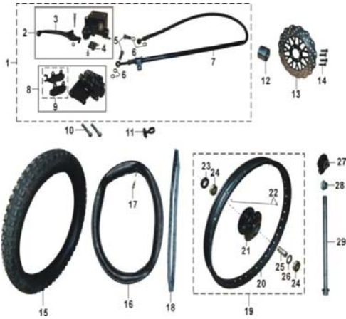
B06 = 前轮 & 前刹车 / FRONT WHEEL & BRAKE ASSY / RUEDA DELANTERA Y FRENO DELANTERO
