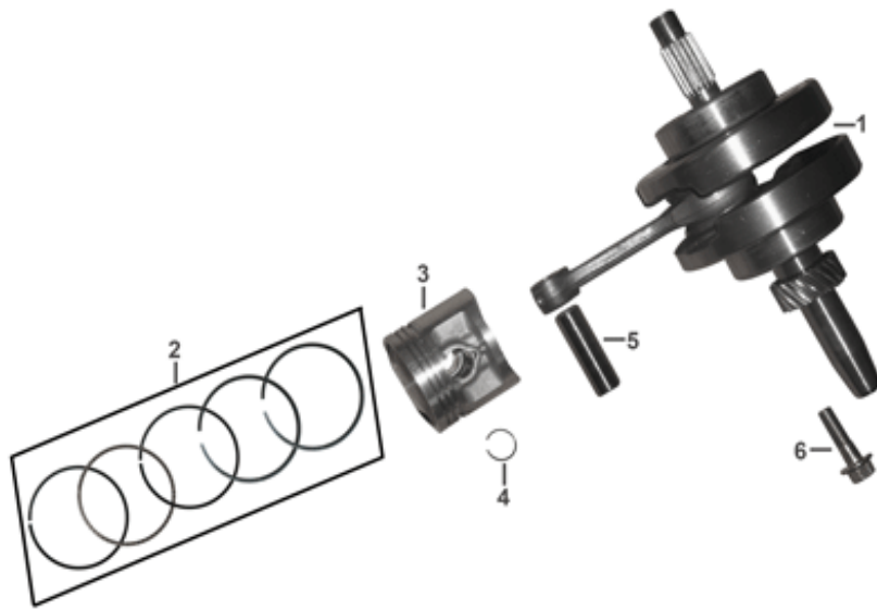
E05 = 曲轴 & 活塞 / CRANKSHAFT & PISTON / CIGÜEÑAL, PISTON Y ANILLOS
