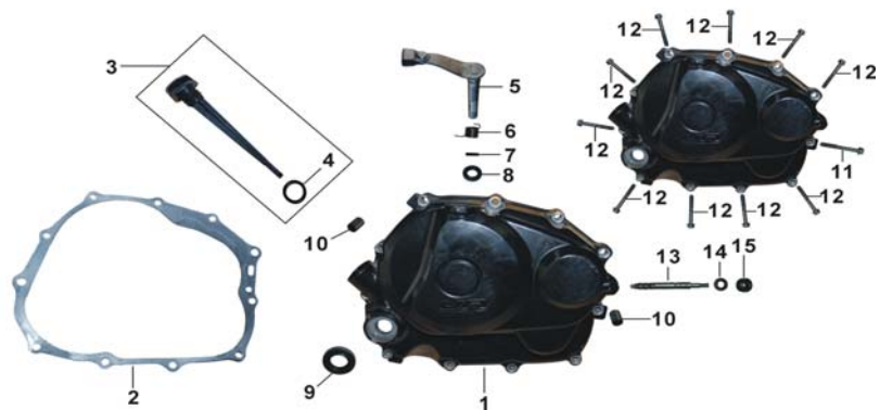
E09 = 左曲軸箱 / LEFT CRANKCASE COVER / CUBIERTA IZQUIERDA DE MOTOR
