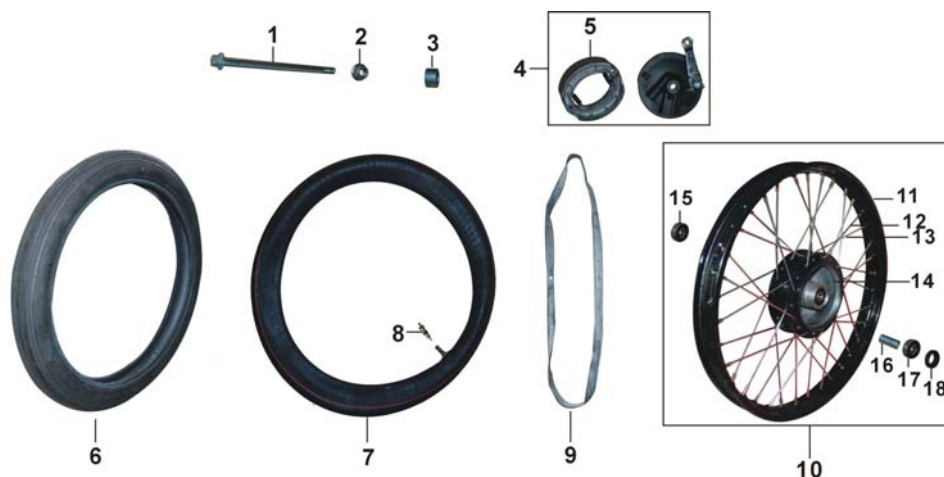
B06 = 前轮 & 前刹车 / FRONT WHEEL & BRAKE ASSY / RUEDA DELANTERA Y FRENO DELANTERO
