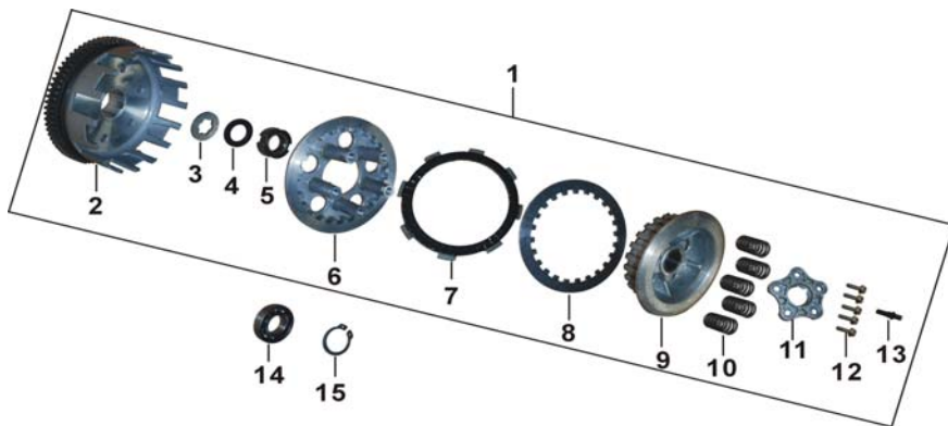
E03 = 离合器 / CLUTCH / EMBRAGUE
